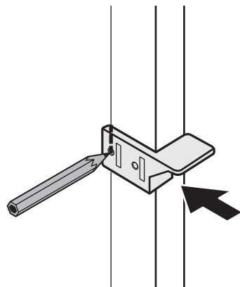
Guía (accesorio para el posicionamiento)
