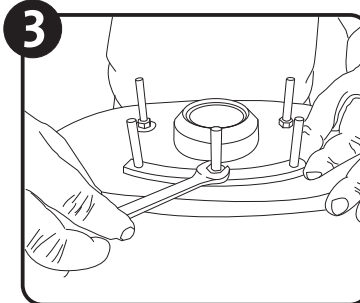
Qty 2 - 5/16-18 bolts to attach metal bracket to bowl 2 Tornillos de 5/16 X 2" fijos a la platina
